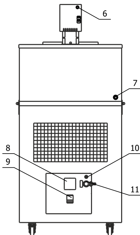
Рисунок 5 — Задняя панель термостата
